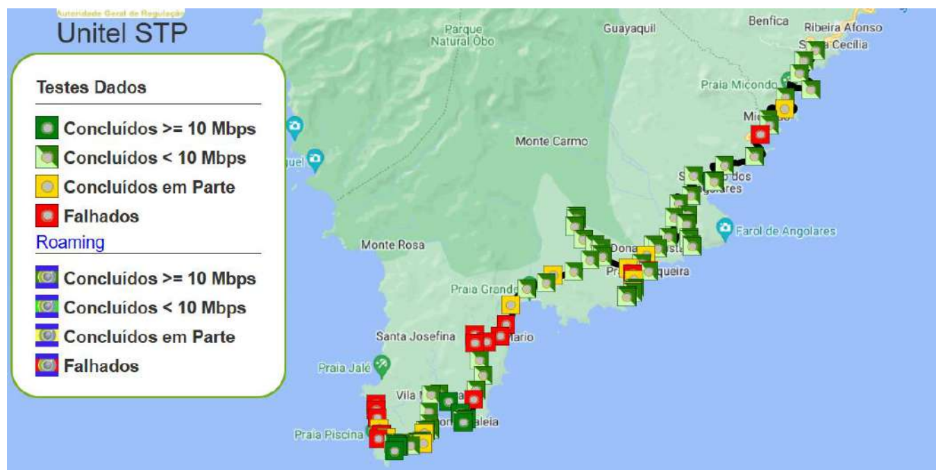
Figura 18 - Mapa de testes de dados efetuados na Rede Móvel UNITEL-STP
