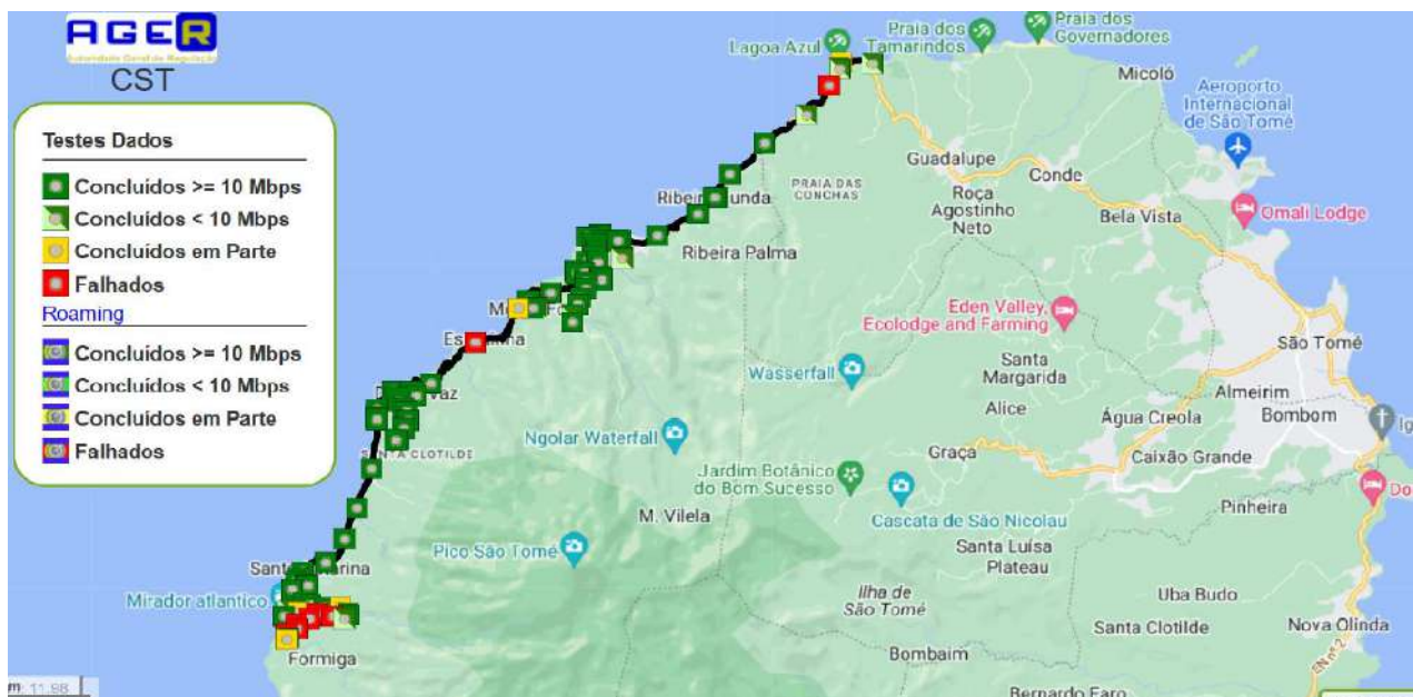
Figura 17 - Mapa de testes de dados efetuados na Rede Móvel CST
