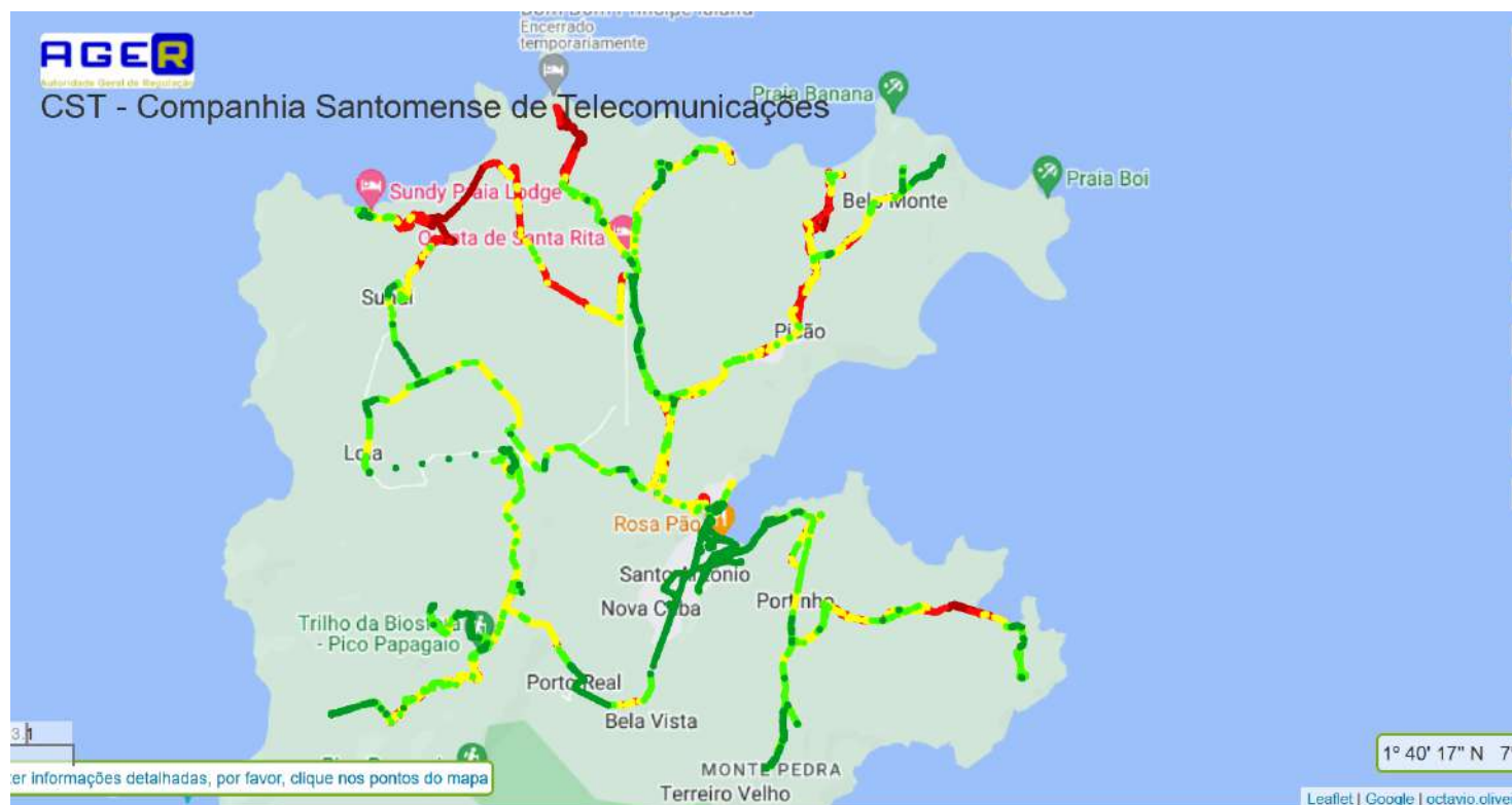
Figura 12 - Cobertura Rede Móvel CST
